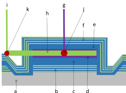
Figura 1. Esquema de la estructura y la operación del microtermómetro: (a) sustrato masivo, (b) estructura DBR, (c) Lámina compuesta de un material de bajo índice de refracción que permita guiar la luz emitida por los nanohilos o microhilos (d) nanohilo o microhilo; (e) Lámina depositada tras deposición de nanohilos o microhilos, compuesta de un material de bajo índice de refracción que permita guiar la luz emitida por el nanohilo o microhilo; (f) estructura DBR tras deposición de nanohilos o microhilos; (g) láser de excitación; (h) luz guiada por el nano- o microhilo; (i) posición del objetivo para recolectar la luz guiada; (j) punto de excitación del microhilo; (k) punto de recolección.
