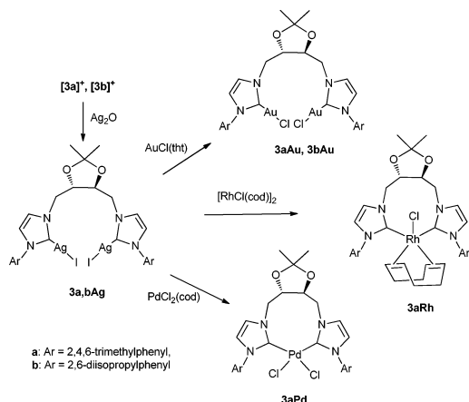
Scheme 2 Synthesis of bis -NHC-complexes
