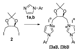
Scheme 1 Synthesis of chiral bis -NHC ligand precursor.
