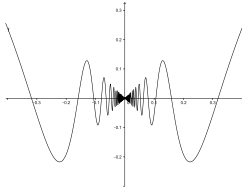
Función x \sin(1/x) .
