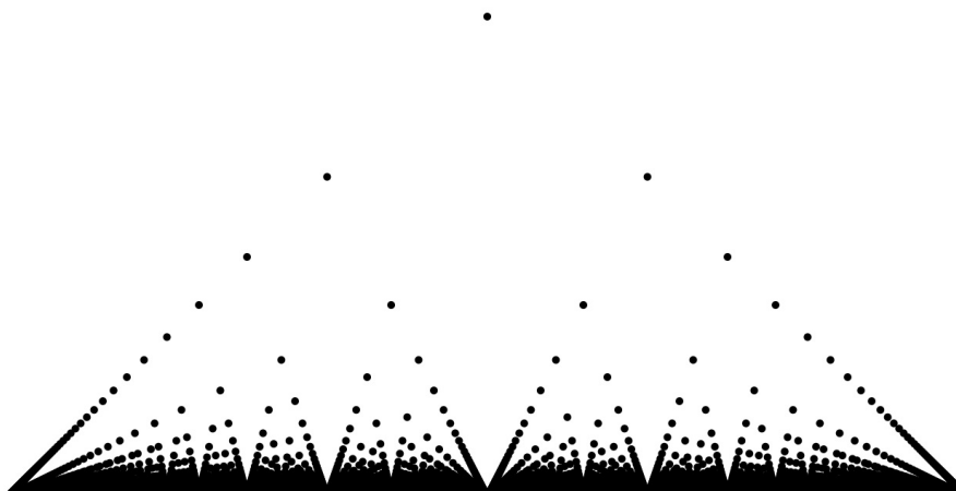
Función de Thomae en (0,1) (dibujo de Smithers)
