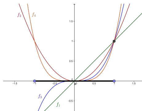
Gráfica de los cuatro primeros términos de la sucesión anterior.
