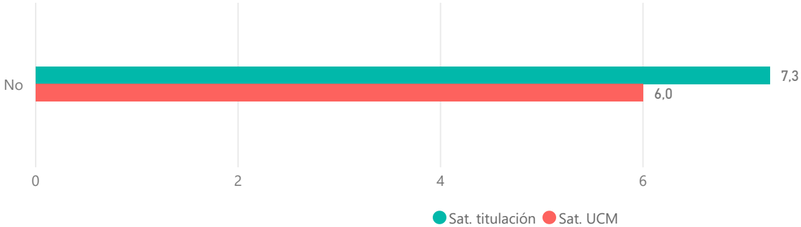
Satisfacción global con UCM y titulación según estancia en el extranjero (valoración en escala 0 - 10)
