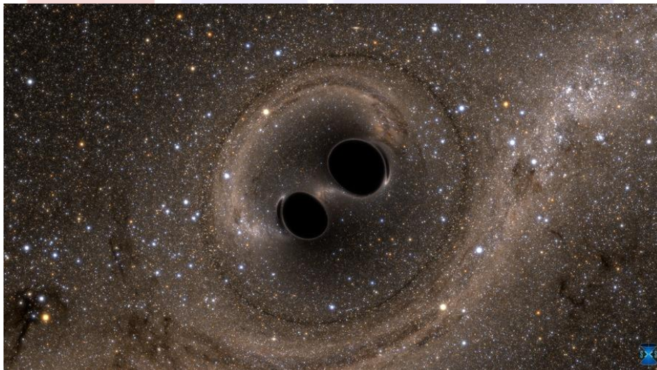
LIGO ha detectado, por primera vez en la historia, la colisión de dos agujeros negros, como se simula en esta ilustración. La fusión de ambos cuerpos ha generado ondas gravitacionales que han sido captadas por los instrumentos de LIGO. / SXS .
