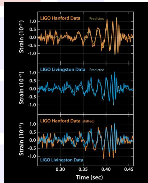
Estos gráficos muestran las señales de las ondas gravitacionales detectadas por los observatorios LIGO en Livingston y Hanford (EEUU). / LIGO .
