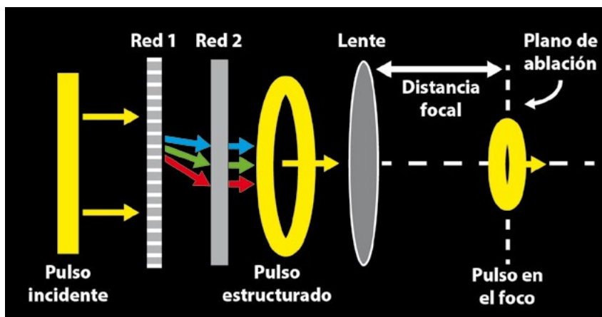
Figura 2.- Dispositivo programable para controlar la distribución espacial de los pulsos en el plano del foco (plano de ablación).
