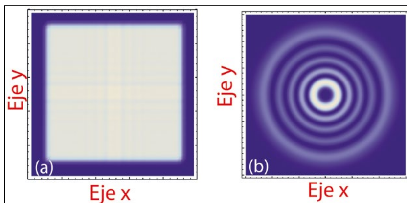
Figura 3.- Simulación de la distribución espacial de pulsos ultracortos generados con el dispositivo programable. (a) Pulso supergaussiano espacial, y (b) pulso con momento angular orbital.
