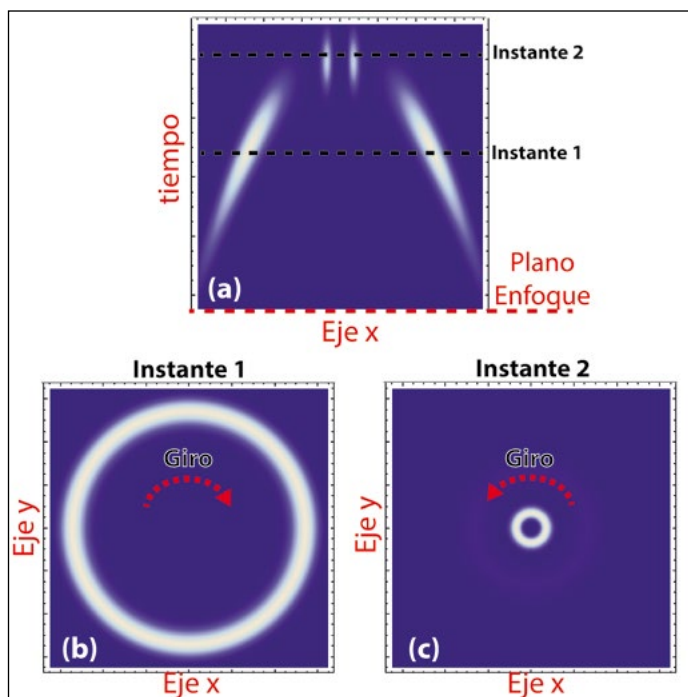
Figura 4.- Diseño espacio-temporal de un pulso con momento angular no-estacionario. (a) Evolución espacio-temporal. (b)-(c) Distribución espacial en el foco en dos instantes distintos
