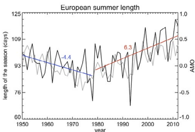
Figura 1. Serie de la duración (en días) del verano europeo (negro) y de la AMO (gris) desde 1950 a 2012. Las tendencias temporales de la duración del verano para los periodos 1950-1978 y 1979-2012 obtenidas mediante una regresión lineal se indican en azul y rojo, y alcanzan valores de -4.4 y 6.3 días por década, respectivamente.
