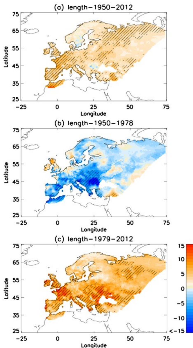
Figura 2. Mapa europeo con los cambios de la duración del verano (expresados en días por década) para el periodo: a) 1950-2012; b) 1950-1978; c) 1979-2012. Las regiones rayadas indican zonas donde los cambios obtenidos mediante una regresión lineal son estadísticamente significativos al 95% de confianza (figura adaptada de Peña-Ortiz et al. (2015)* ©American Meteorological Society. Used with permission).
