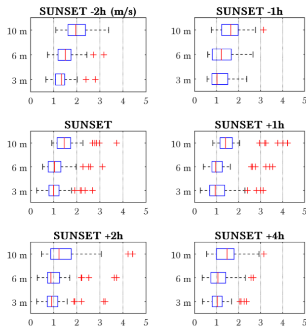
Fig 2. Diagramas de caja de la variación de la velocidad del viento en los niveles de 3, 6 y 10 m en los eventos catabáticos, para diferentes horas relativas a la puesta de sol. La línea vertical roja de las cajas representa la mediana de la distribución, la caja azul delimita q_1 y q_3 (los cuartiles 1 y 3 respectivamente), los whiskers (líneas negras que salen de las cajas) indican los valores extremos no considerados outliers , y los outliers (cruces rojas) se dibujan para valores mayores que q_3 + 1.5(q_3 - q_1) y menores que q_1 - 1.5(q_3 - q_1) .
