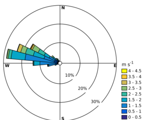
Fig 1. Rosa de vientos a 10 m durante las 2 horas posteriores al establecimiento del flujo catabático en La Herrería en el periodo [22/06/2017 - 26/09/2017].
