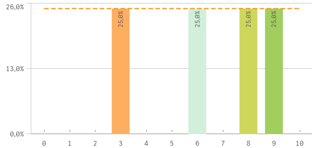
Prácticas
