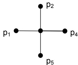
Figura 2. Una estrella o ejes con cinco puntos
