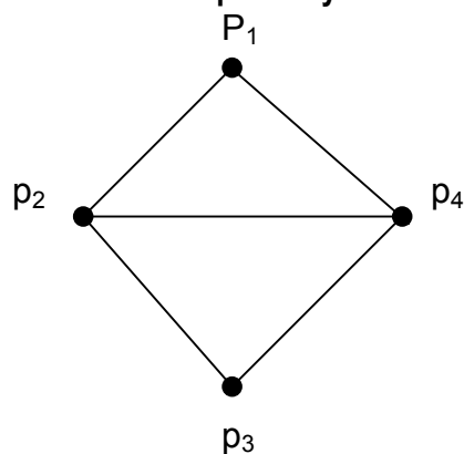
Figura 4. Un grafo con cuatro puntos y cinco aristas
