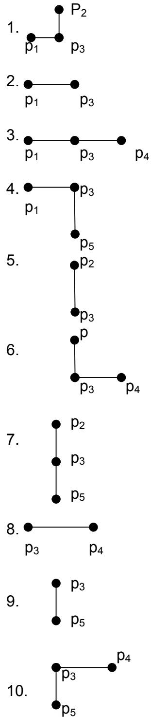
Figura 3. Las diez geodésicas del grafo de la Figura 2
