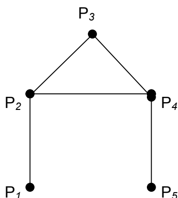
Figura 1. Gráfico con cinco puntos
