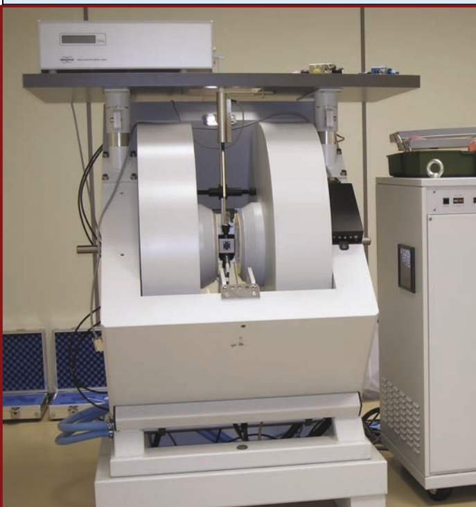
BRUKER EMX-10/12 0-0.4 Tesla
