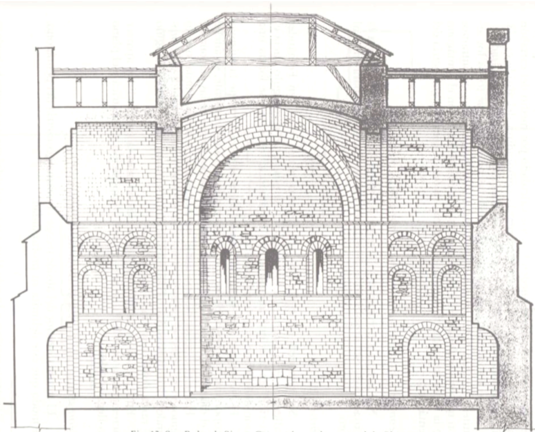
Fig. 13. San Pedro de Siresa. Geometría en el arco toral de Chueca.
