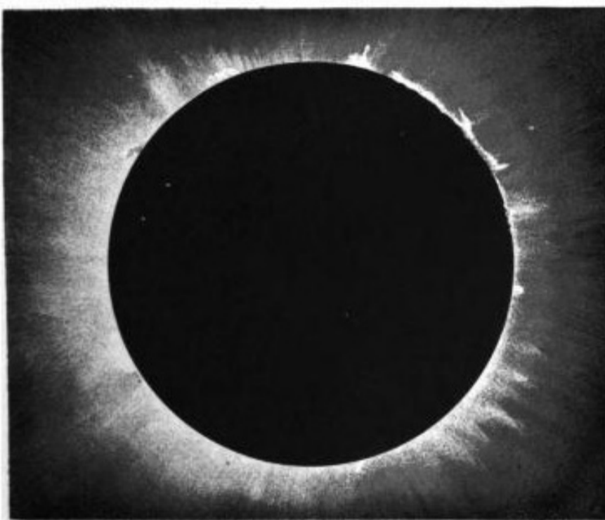
ÉCLIPSE TOTALE DE SOLEIL
