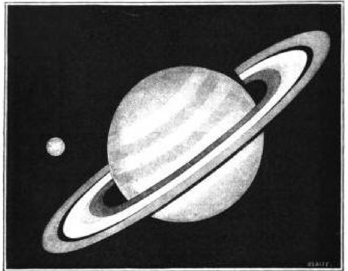
Fig. 92. — Saturne et la Terre; dimensions comparées.
